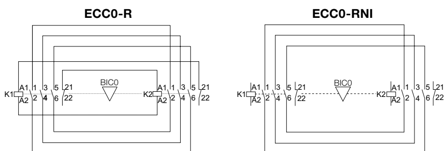
Diagramas elétricos
