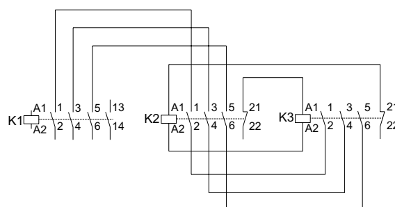
Diagrama elétrico
